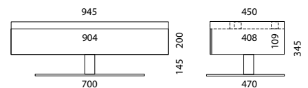
DS03 Passend für Bose CineMate 1SR, CineMate 130 und Lifestyle 135 (ohne Subwoofer-Unterbringung im Möbel) Klappe (Glasfront) und Ablage für Bose Sound Projektor
