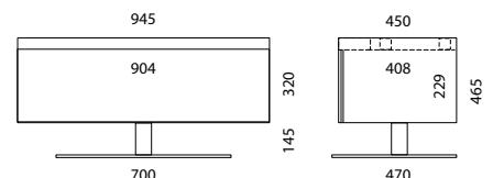
DS04 Passend für Bose CineMate 1SR, CineMate 130 und Lifestyle 135 (mit Subwoofer-Unterbringung im Möbel) Stoffbespannte Klappe und Ablage für Bose Sound Projektor
