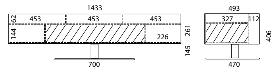
DS51 Passend für SPECTRAL Soundsysteme BRA2 und SCA3 Stoffbespannte Klappe, 3 Gerätefächer oben, 3 Fächer unten (1 Fach für Soundsysteme, BRA2 oder SCA3 müssen eingesetzt werden)
