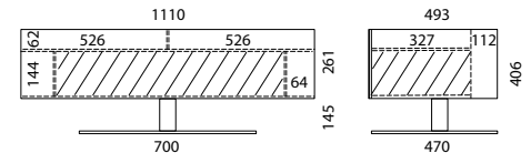
DS81 Passend für SPECTRAL Soundsysteme BRA2 und SCA3 Stoffbespannte Klappe, 2 Gerätefächer oben, unten 1 Fach für Soundsysteme (BRA2 oder SCA3 müssen eingesetzt werden)
